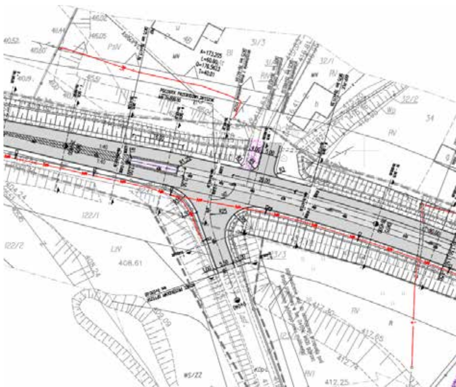
Projekt przebudowy skrzyżowania Maciejowa-Czaczów-Barnowiec
